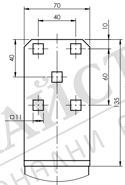
SZCZEGÓŁA A SKALA 2:5
