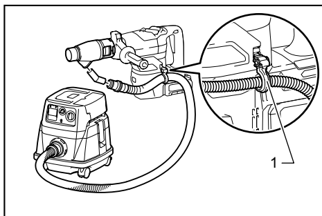
► 1. Hose holder
