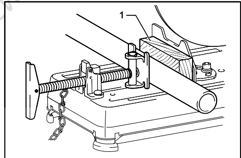
► 1. Spacer block
